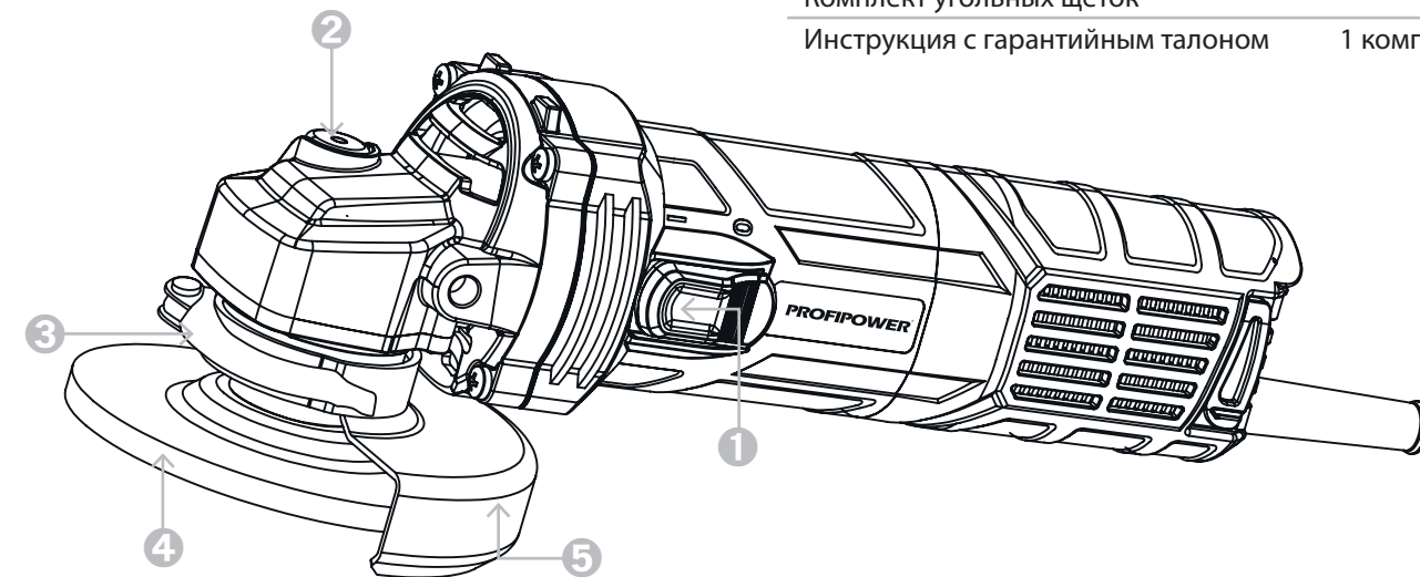
Рисунок 1.5. Устройство изделия
