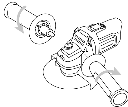
Рисунок 2.2.1. Установка дополнительной рукоятки
