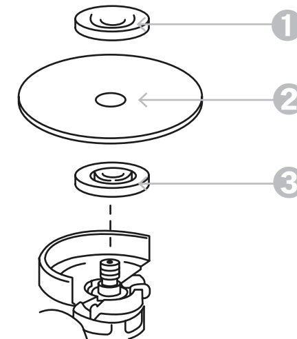
Рисунок 2.2.4. Установка оснастки
