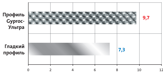
Сравнительные тесты удержания самонарезающего шурупа в гладком металле и в металле профиля Гуррос-Ультра
